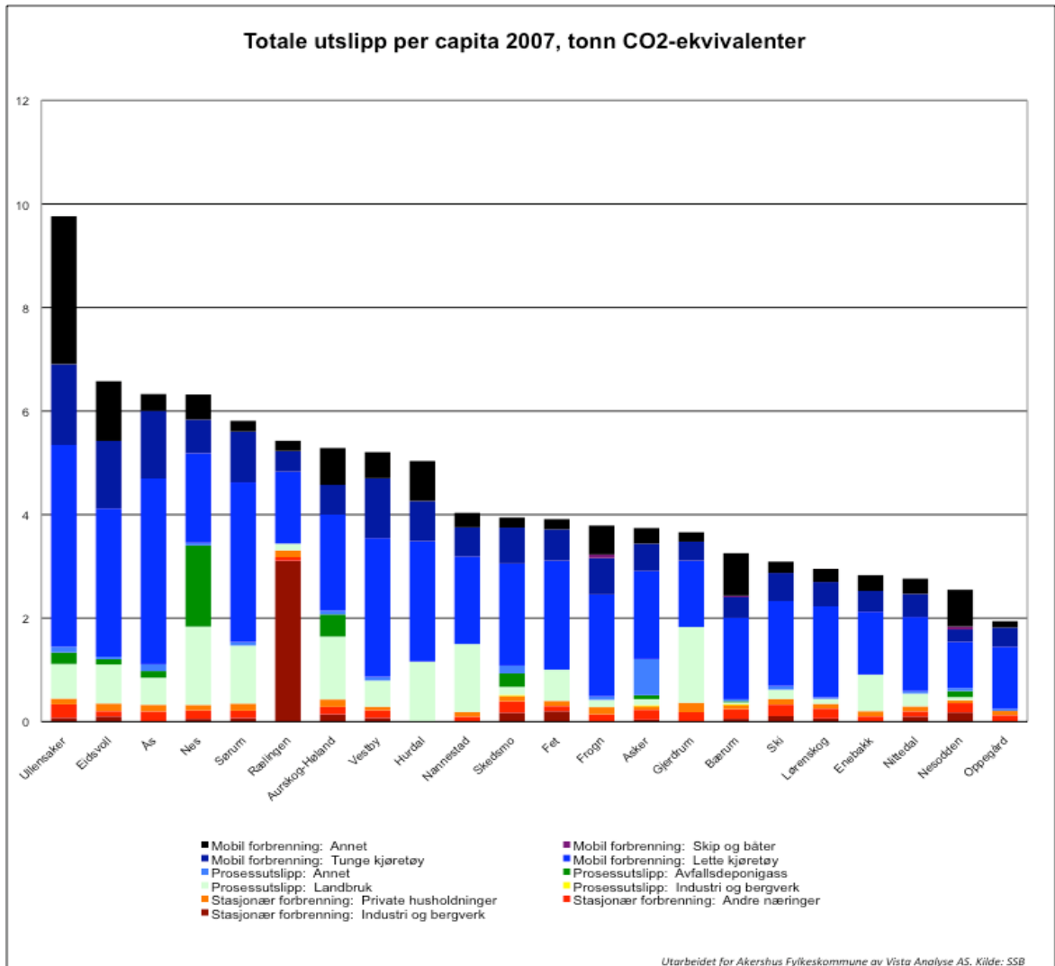
Figur 5 - Utslipp av klimagasser (CO2-ekvivalenter) i Akershus i tonn per innbygger i 2007 fordelt for kommune og sektor. Kilde: SSB/KLIF.
