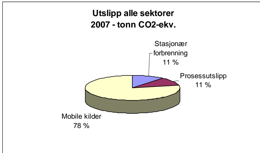
Figur 3 - Sektorfordelt utslipp for 2007. Kilde: www.klif.no .
