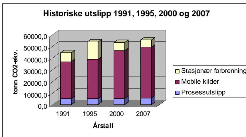
Figur 2 - Historiske utslipp av CO2-ekvivalenter fra 1991-2007. Kilde www.klif.no .
