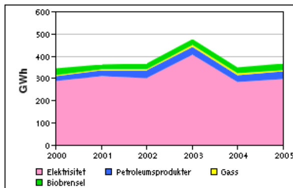
Figur 7 - Utvikling i bruk av energibærere. Kilde Hafslund LEU
