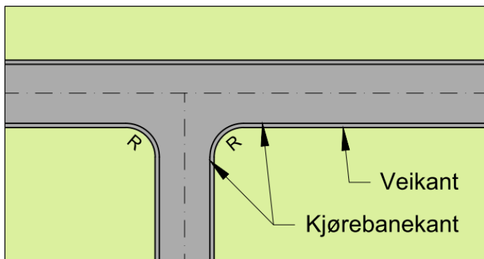
Figur 5.28: Tilstutningsradier mellom kjørebane kantene i et veikryss
