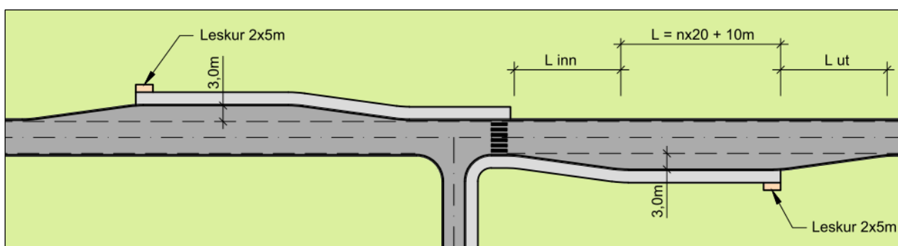
Figur 5.41: Utforming av busslomme
