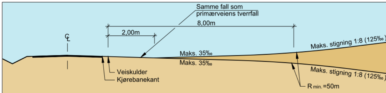
Figur 5.31: Tillatt lengdeprofil for boligvei i veikryss
