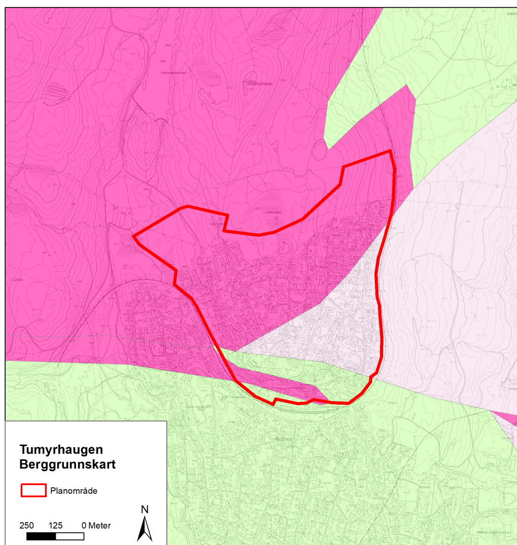
Figur 3 Planområdet lagt oppå berggrunnskart der rød farge i nordvest er kalkfattig normarkitt, mens grønne farger er kalkrike bergarter av kambrisk alder, lys fiolett i øst er gneis. ( http://geo.ngu.no/mapserver/berggrunnWMS ).
