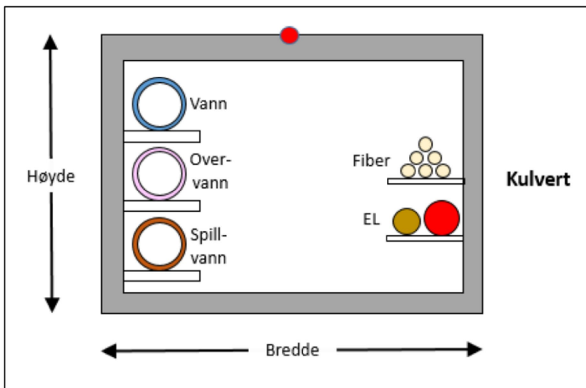
Figur 10. Eksempel kulvert
