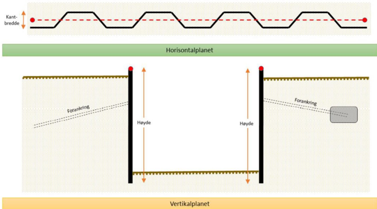
Figur 11. Eksempel på stedefesting av vertikal spuntvegg i horisontal- og vertikalplanet
