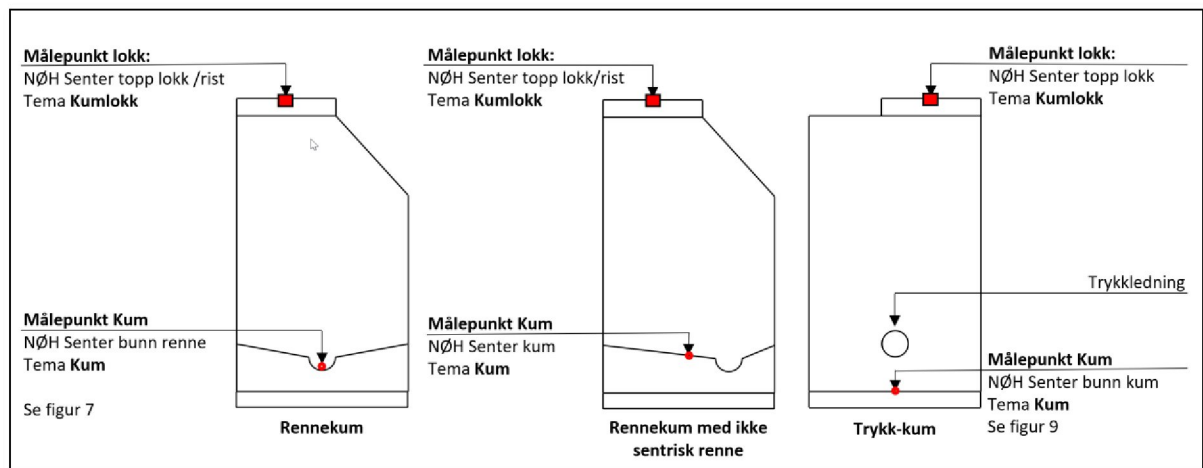
Figur 1. Hvordan måle inn installasjon med lokk
